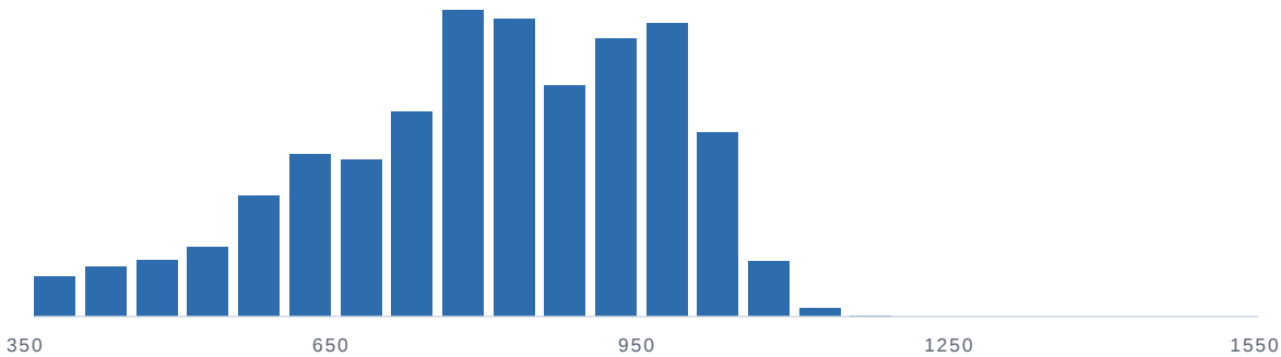
35トレード系列のブートストラップ総損益分布（10万回）
